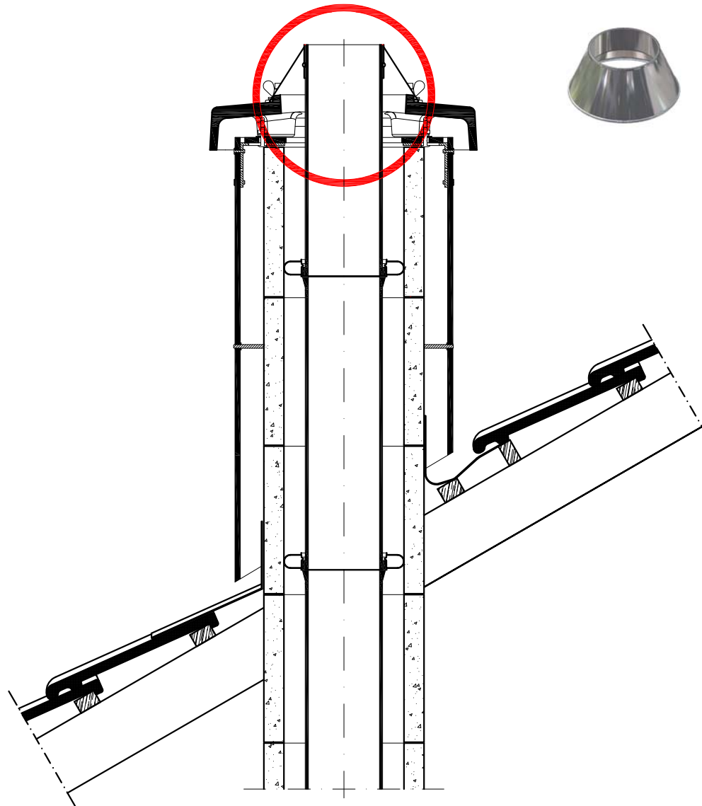
Abströmkonus
