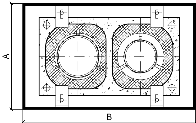
Draufsicht ohne GFB-Abdeckplatte
